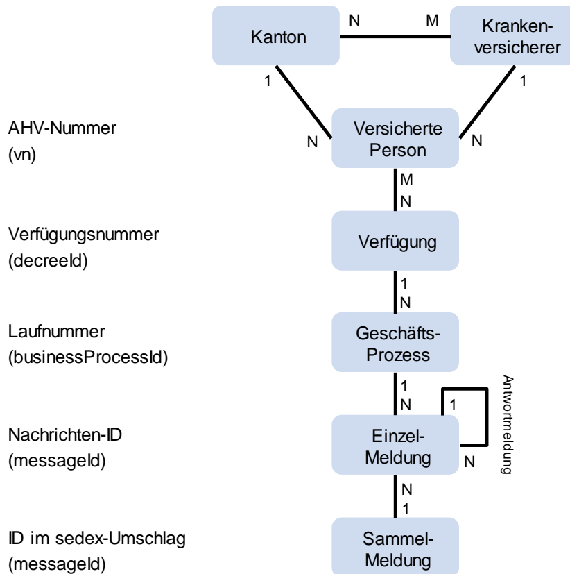
Abbildung 11: Datenmodell
